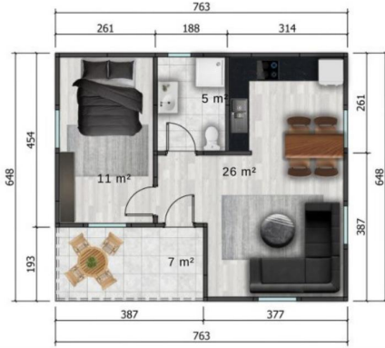
Kat planı / Floor plan
